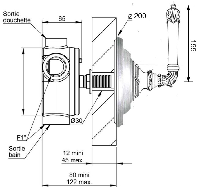
Montage sur cloison
