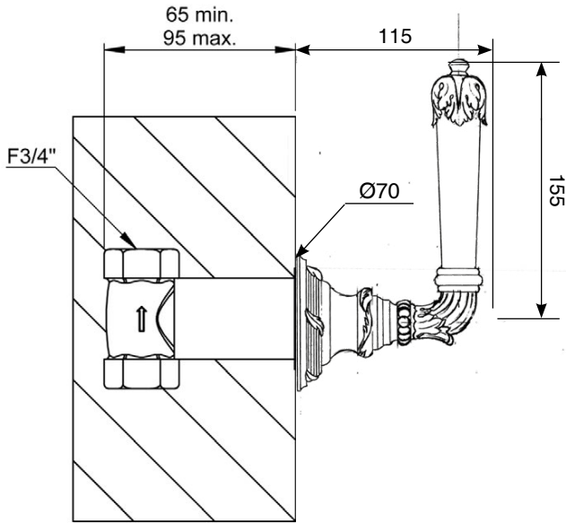
Montage par scellement
