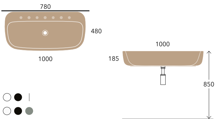
Monò 100 art. MN100L
