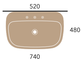
Monò 74 art. MN74L
