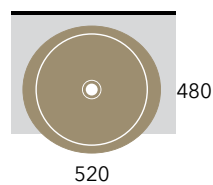
Fonte Tonda art. FT52L
