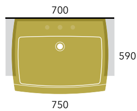
Una 75 art. UNA75L
