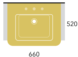
Volo 66 art. VL66L
